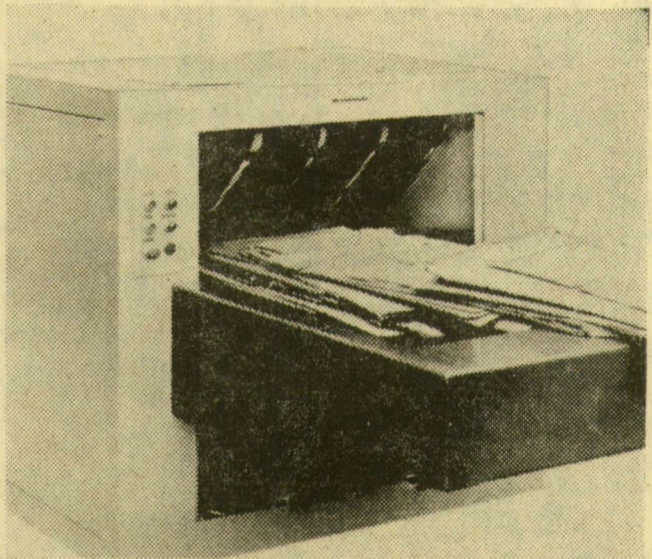
„IRATEVŐ”. A francia Manuteir gyár érdekes „iratevő” gépet szerkesztett, amely óránként 1,2—6 tonna papírt képes apróra szelgetni. A gépet nagy irodákban, levéltárakban hasznosítják, a főlöslegessé vált irathalmaz megsemmisítésére
