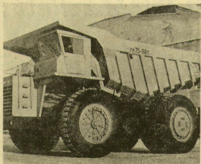
SZOVJET ÓRIÁS. A Szovjetunióban a hatalmas méretű földmunkákhoz új és új nagyméretű munkagépek készülnek. Képünk a legújabb „Belaz-549” nevű óriás dömpert mutatja be, amelynek hat kereke van, s motorja több száz lóerős. A legmeredekebb emelkedőn is képes terhét elszállítani
