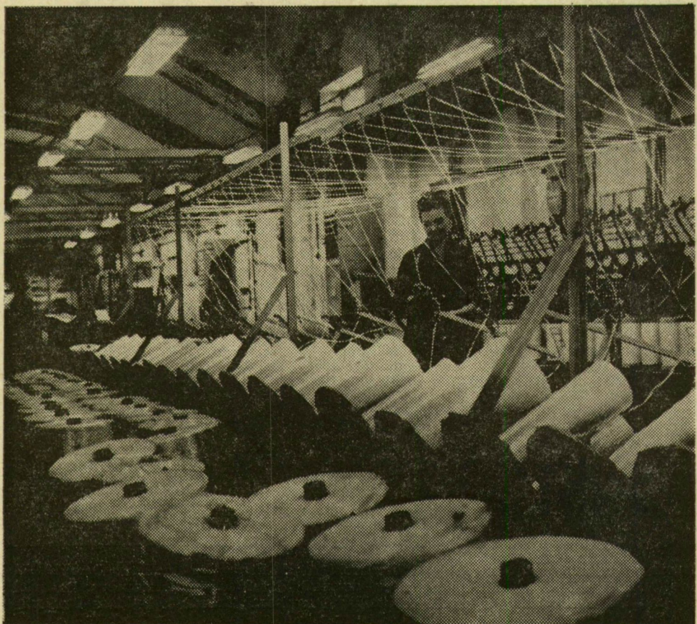
MŰANYAG A KENDERIPARBAN. A Kenderfonó és Szövőipari Vállalat újszegedi központi gyárában már két darab Covema-gépsor dolgozik. Képünk egy nagy teljesítményű sodrógépet ábrázol, amelyen a polipropilén szálakat sodorják össze erős zsineggé
