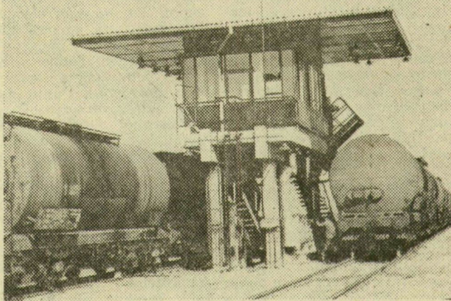
Az algyői szénhidrogén medencében a szállítások meggyorsítására központi vasúti olajtöltő állomás épült. Itt tízpercenként töltönek meg egy-egy tartályvagont és naponta indulnak a hosszú szerelvények.
