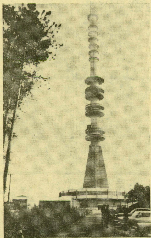
ÉPÜL AZ ÚJ TV-TORONY. A kelet-nyugati mikroánc utolsó — nyugati láncszeme — a 135 méter magas tv-torony építése rövidesen befejeződik Sopronban. Az URH normál és színes televíziós közvetítések, valamint az első lépésben 480 egyidejű telefonbeszélgetésre alkalmas berendezés monumentális vasbeton tornyát december végén adják át az építők.
