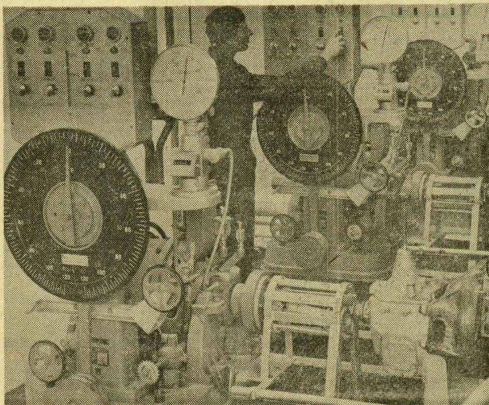
MOTOROK A VIZGÁLÓPADON. A Szegedi Autójavító Vállalat új üzemében korszerű műszerekkel ellenőrzik a megjavított gépkocsimotorok működését, s csak utána építik be az alvázakba. Képünk a motorok biztos vizsgáztatóját, a nyomaték-mérő fékpadokat mutatja be
