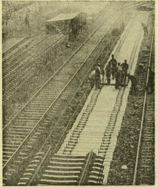
ÚJ VASÚTI PÁLYA. Budapest és Miskolc között épül meg az ország legkorszerűbb vasúti pályája. A korszerű vasútvonal lehetővé teszi majd, hogy a vonatok 140 kilométeres utazósebességgel közlekedhessenek. Jelenleg Miskolc és Nyékládháza között dolgoznak az építők, s ez a szakasz még ebben az évben elkészül. Képünkön: a felső-szolcai telephelyen korszerű módszerekkel előre összeszerelik a pályatest egyes elemeit
