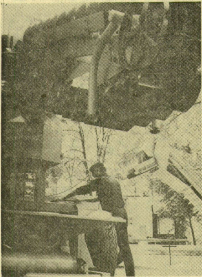
KORSZERU AROKASO. A lengyel nehézipar új rendszerű árokásó gépet gyárt, amelyet a hagyományos megoldással ellentétben végtelenített láncsorra szerelt marófejekkel készítenek. A gép nemcsak árkot ás, hanem a kánalaival kimarkolt földet egy tartályba továbbítja, majd az út szélére lerakja.
