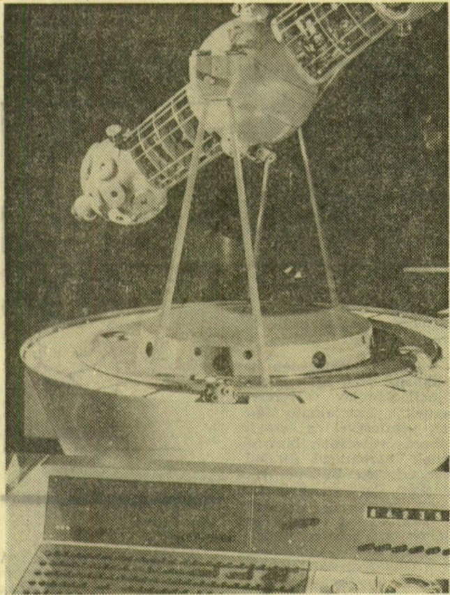
PRÓBAPADON A MŰHOLD. Mielőtt egy-egy távközlési mesterséges holdat a világűrbe küldenének, hosszú, rendkívül gondos ellenőrzésnek vetik alá. Képünk egy amerikai, televíziós közvetítésekre alkalmas mesterséges hold próbapadról készült, amelyen mintegy 200 féle „műhold-funkciót” ellenőriznek. A vizsgálati eredményeket magnetofonszalagra rögzítik.
