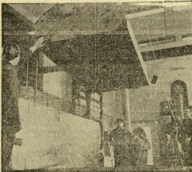
A rönkhasító szalagfűrészes új, korszerű, olasz gyártmányú berendezés. Ebből a hatalmas mahagóni rönkből hasít furnérlemezeket a Béke II-es szocialista brigád irányításával
