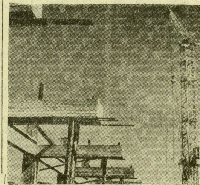
Szeged jelenlegi legmagasabb építőipari daruja a Budapesti út melletti, új tejjüzem építésénél dolgozik. Nemrég érkezett Lengyelországból. A hatalmas, negyven méter magas daruval kényelmesen emelik helyükre a több tonnás, előregyártott betonlemezeket is.
