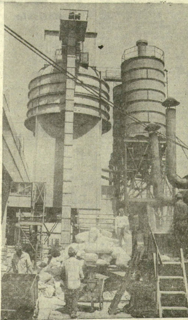
Szeptember 1-én már egyes részlegeiben próbaüzemel a ferencvárosi házgyár. Az automatikusan működő, nagyteljesítményű házgyár a tervek szerint január elsejétől már teljes kapacitással dolgozik. Képzünk: Részlet az épülő házgyárból
