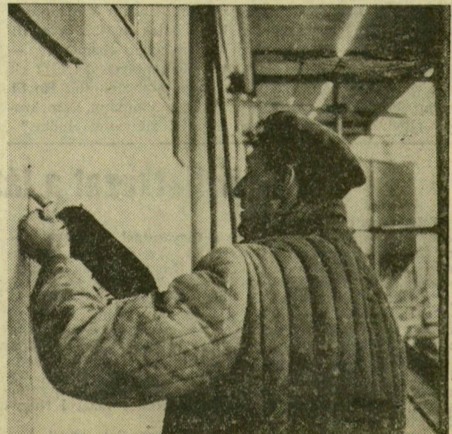
Több emelet magasságban palnakított műanyagpalattákkal töltik a homlokzat hézagait
