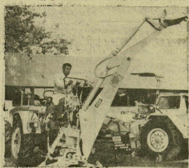
Magyar és nyugatnémet gépek „házassága”: a Schaeff cég olyan munkagépet mutatja be, amelyet magyar gyártmányú erőgéppel kapcsol össze. U-28-as traktorra HT-5 típusú hidraulikus mélyásó- és rakógépet kapcsolnak
