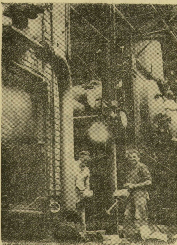
Téglával falazzák a II-es számú kazán tűzterét
