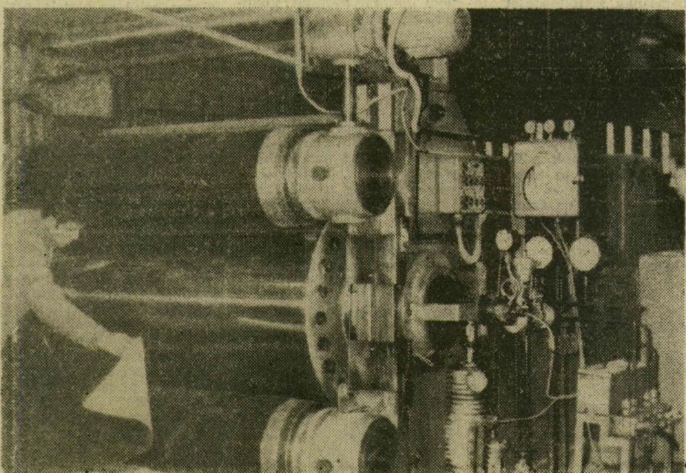
Munka közben a cseh gyártmányú folyamatos vulkanizálógép
