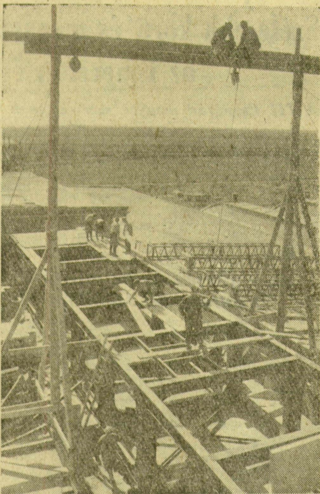
A korom-bunker — nyersanyag tárolásra használják majd, a gyártás megkezdésekor — acélszerkezetének szerelése
