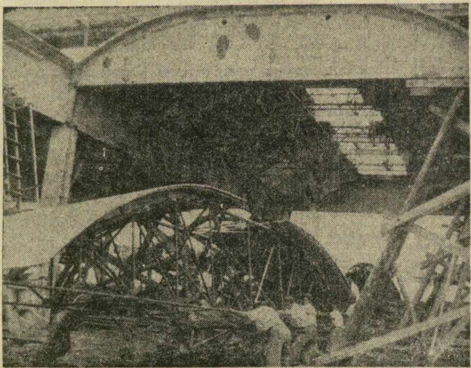
Az épülő Szegedi Műszaki Gumigyárban már harmadik hete készítik a nagyeszernök hejlesztését. Képünkön az ácsolatot helyettesítő vasszerkezet látható, amit a munkások tovább visznek, ha a tető betonja már megkötött
