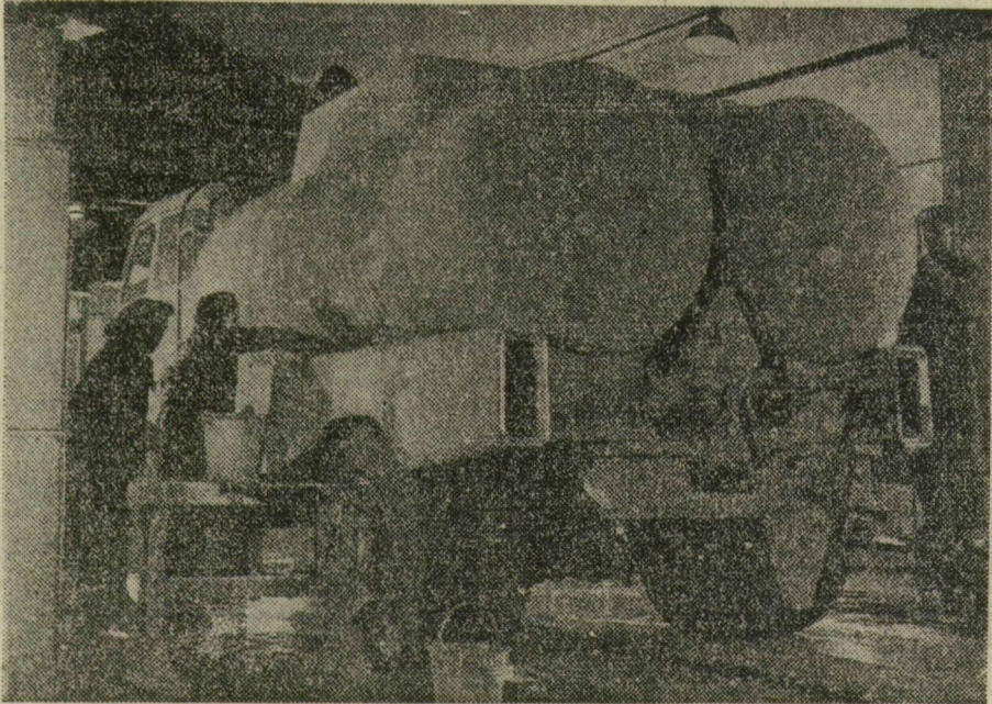
A csepeli autógyárban elkészült a D 707-es anyagszállító gépkocsi prototípusa. A gépkocsi hathengeres, 145 lóerős Csepel motorral készült, s a nyerges vonatokat helyett meredek utakon használható. Tervezője Csefali István mérnök, formatervezője Cserny Miklós grafikus. Az új gépkocsit először az idei lipcsei vásáron mutatják be. A képen: a festőben dolgoznak az új gépkocsin
