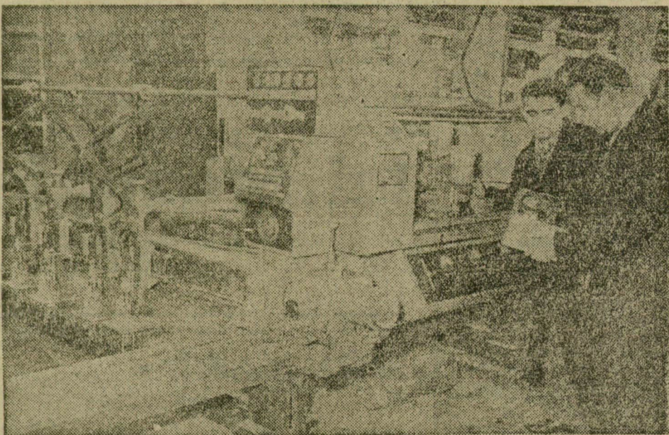
Szeged testvérvárosának, Ogyesszának egyik üzemében automata autogéngvágót szerkesztettek. A fotoelektron masolóval felszerelt automata önállóan követi a műszaki rajz utasításait és egyidejűleg hat alkatrészt képes kivágni az acéllemezből. A gép — melyet Ogyesszáról neveztek el — fél centimétertől 30 centiméter vastagságú anyagokból tetszés szerinti méretekben képes idomokat, alkatrészeket kimetszeni. Az automata kezeléséhez mindössze egy ember szükséges. Képiükön az új automata és tervezői láthatók.
