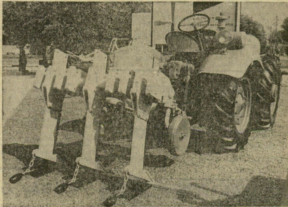
A háromkéses altalajlazító gép talán a legnagyobb érdeklődésre tart számot a munkagépek között. Ahol már alkalmazták ilyen vagy hasonló munkagépet, az idei búzatermés átlagosan 5-6, sőt 8 mázsával lett magasabb.
