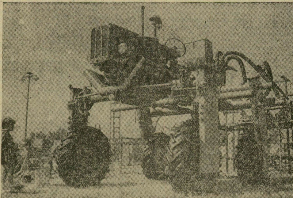
Az idei Országos Mezőgazdasági Kiállításon és Vásáron a szőlő művelő hidas gépek egész kis családját mutatják be. Ezzel az UE-28-as hidas traktorral bármilyen sor- és tökétevélságra beállított szőlőtelepen az összes munkát elvégezhetjük, a metszés és a szüret kivételével. A traktor — amikor a szőlőtelepeken nincs számára munka — vonattalra a szántóföldi talajmunkákra is felhasználható.
