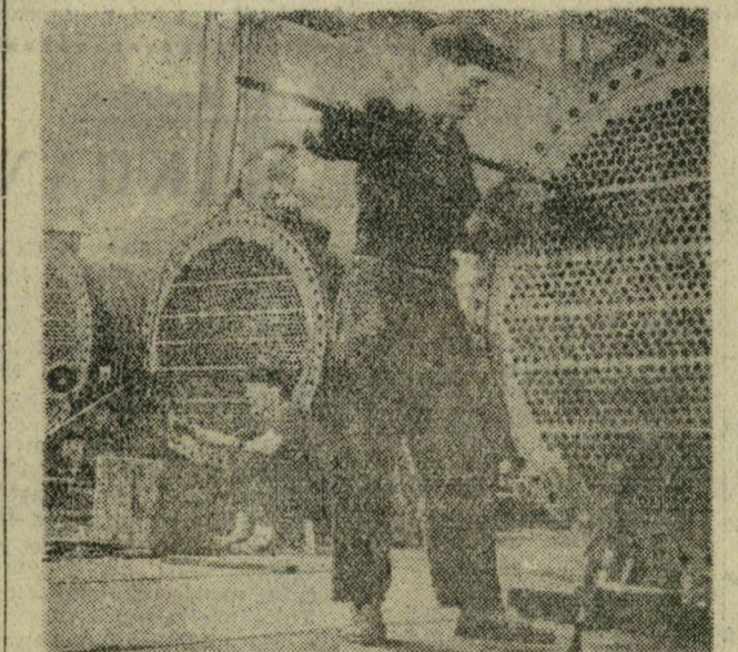
Hőkecsere hővezetések készülnek exportra a budapesti Április 4 Gépgyárban. A vegyipari üzemekben használatos hővezetések közül ebben a negyedévben kilenc darabot készítenek mintegy 4 millió forint értékben.
