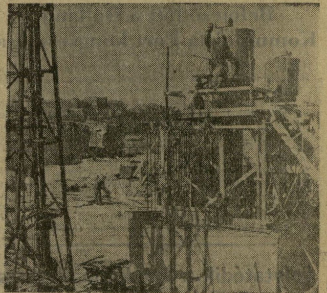
Budapesten nagy ütemben folyik az új Erzsébet-híd felépítése. A pesti oldalon folyó építkezésről készült felvételünk, melyen a munkának azt a mozzanatát látjuk, amint két óriás, 15 méter mély keszont képeznek ki, hogy ezekkel megakadályozzák a hídfő esetleges csuszamlását.
