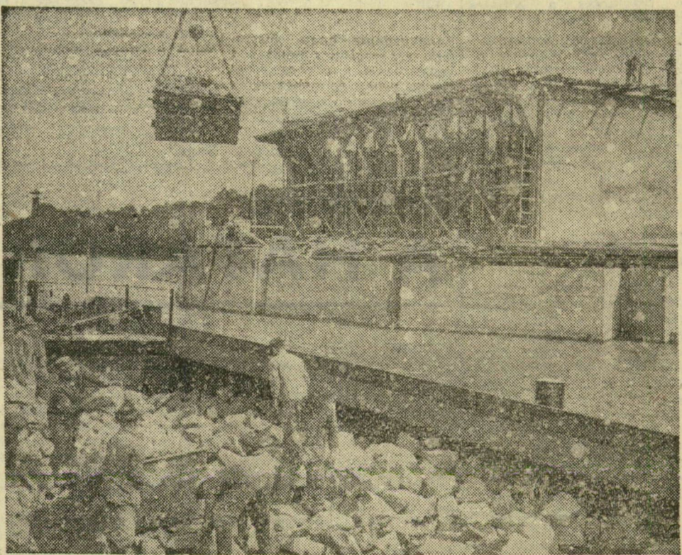
Uszályokon hordják a követ a vízkivételi mű mesterséges szigetének megépítéséhez
