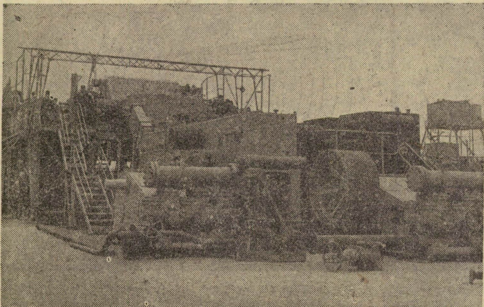
A Ploesti-i »Május 1« üzemekben egy új kőolaj gyorsfűróberendezést gyártottak automatizált kapcsolókkal, 47 méter magas toronnyal. A gyorsfűróberendezés furási mélysége 3200-3500 méter.
